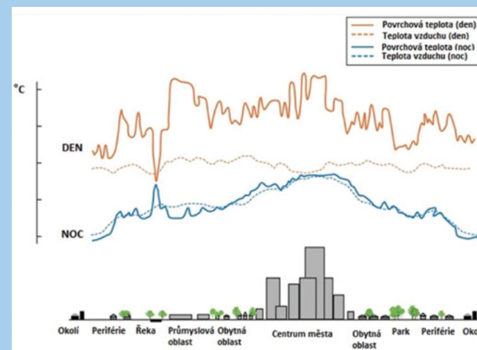
Obr. 2: Městský tepelný ostrov – průběh teplot během dne a noci
