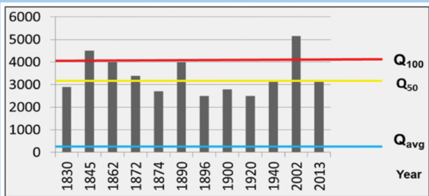
Obr. 7: Povodně na Vltavě v období 1830–2020
